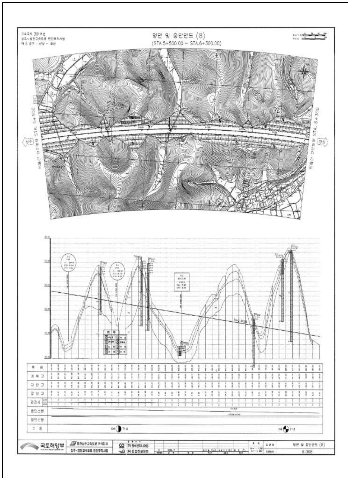
【그림 48.1.4】 평면도
